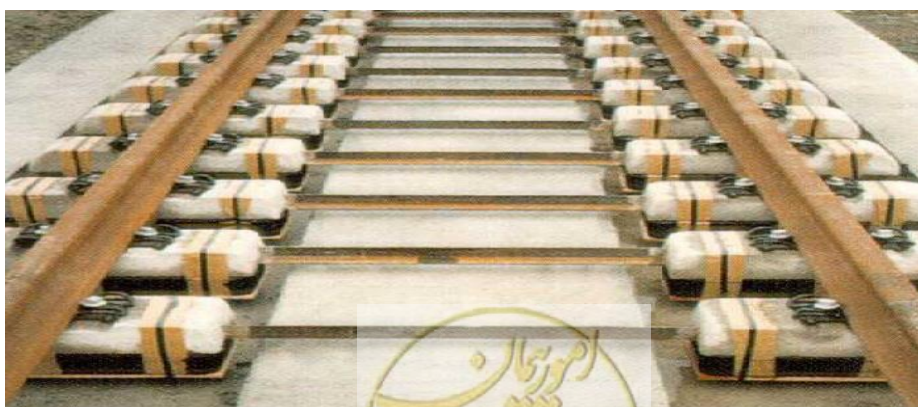
شکل ۲-۱۲ نصب تراورسها در بستر سیستم والو
