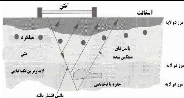
شکل ۲۸-۲ اصول عملیاتی ژئورادار
