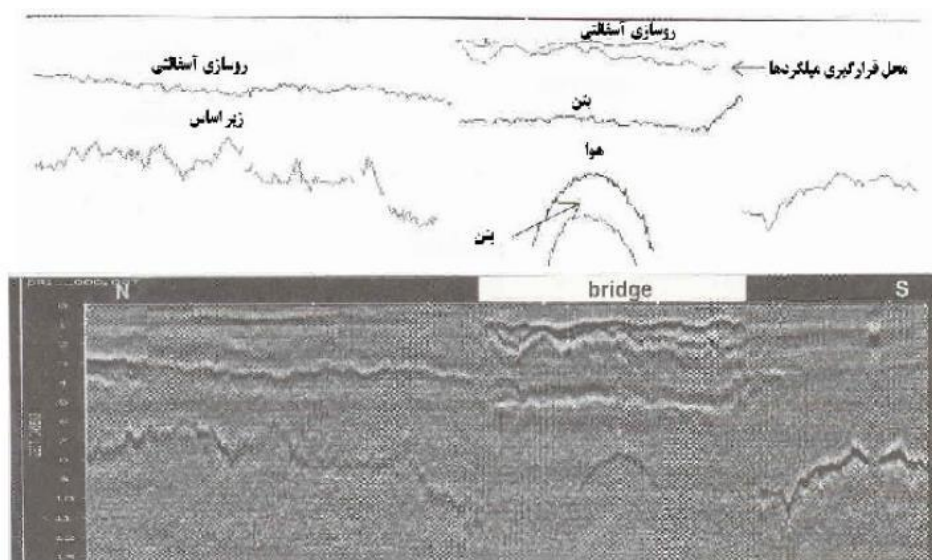
شکل ۲۹-۲ نمایی عمومی از خروجی ژئورادار
