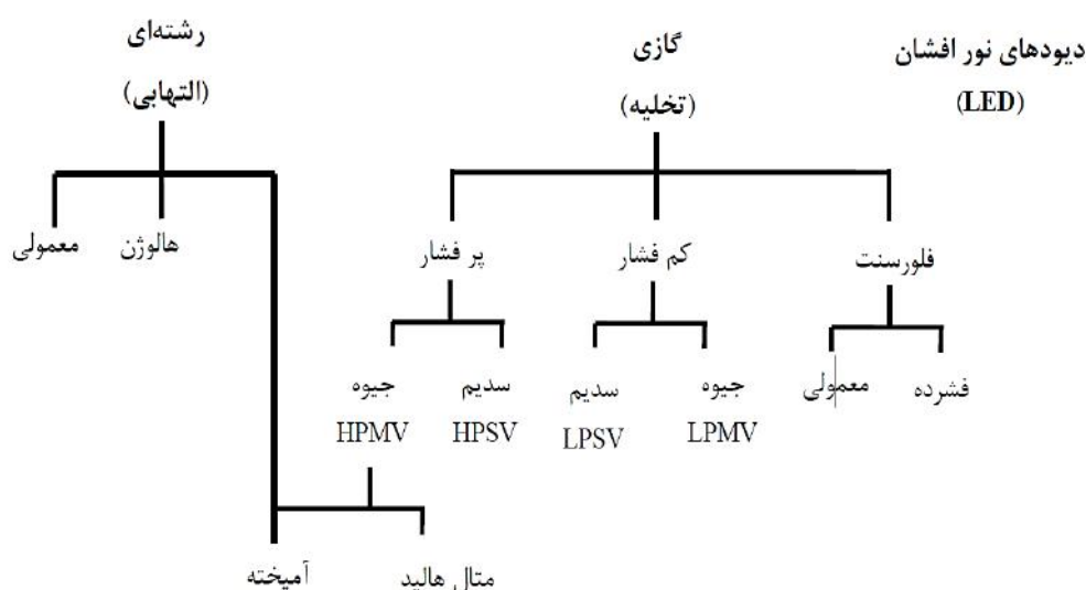
شکل ۳-۳ خلاصه فناوری‌های تولید لامپ
