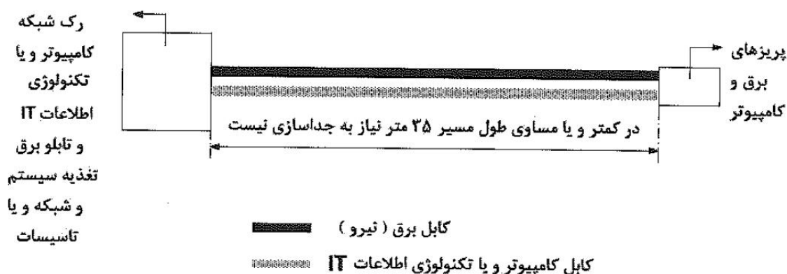
طرحواره مسیر مشترک کابل برق و کابل کامپیوتر یا فناوری اطلاعات IT برای طول مسیر کمتر یا مساوی ۳۵ متر
