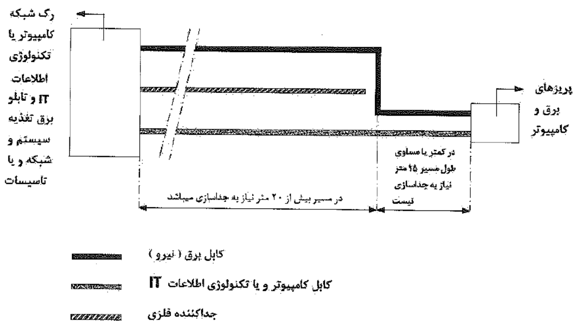
طرحواره مسیر مجزا و مشترک کابل برق و کابل کامپیوتر یا فناوری اطلاعات IT برای طول مسیر بیش از ۳۵ متر
