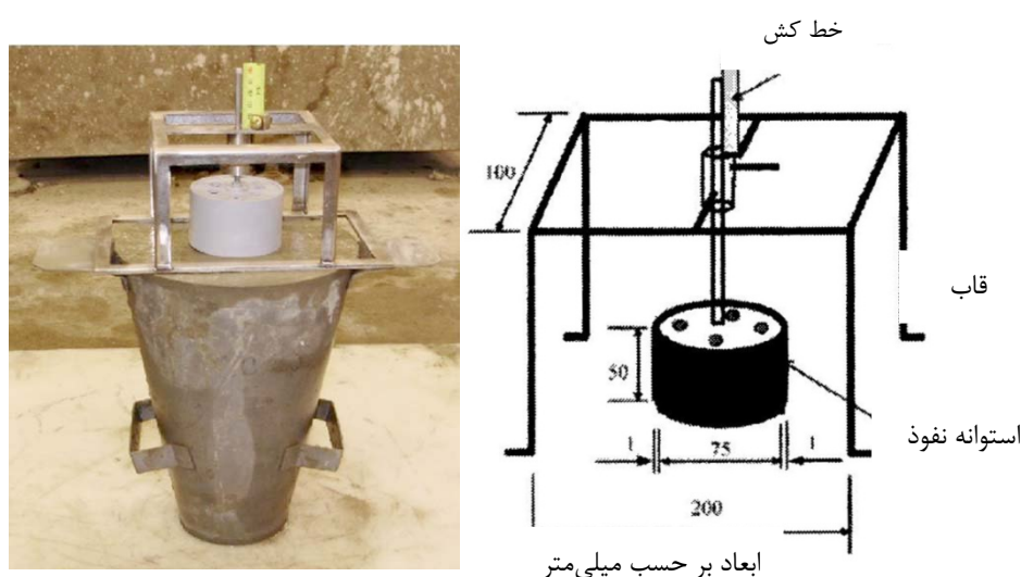
شکل ۳-۱۱ دستگاه نفوذ برای تعیین مقاومت در برابر جداشدگی
