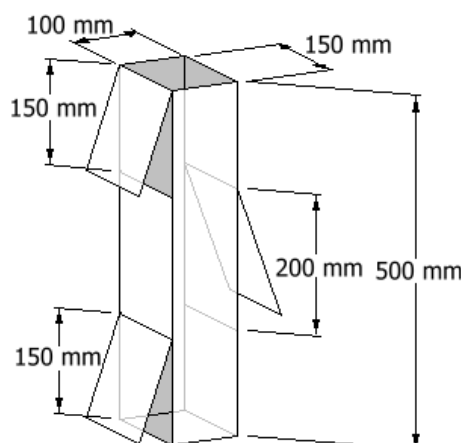
شکل ۳-۱۲ دستگاه آزمایش ستون جدا شدگی دینامیکی [70]
