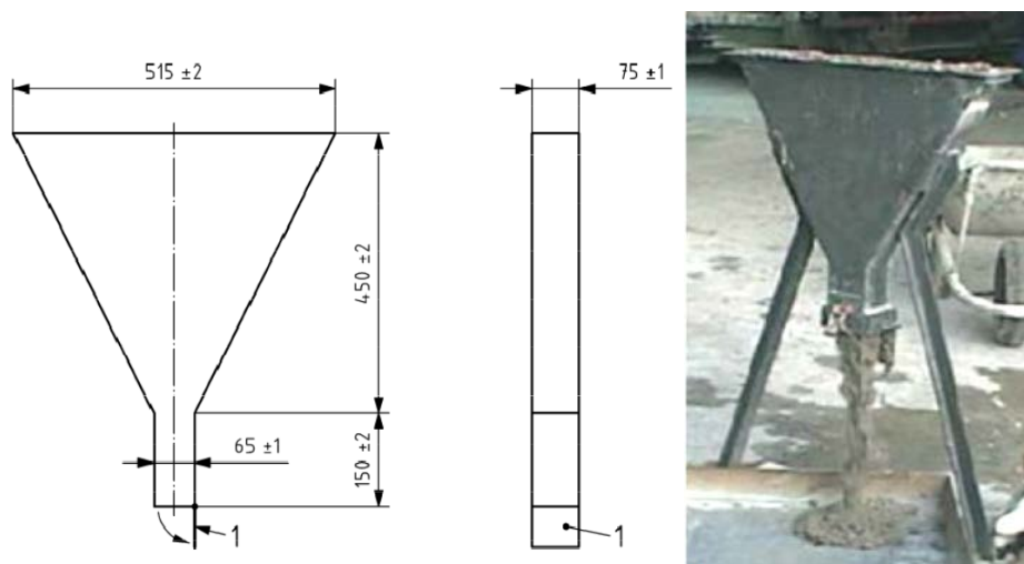
شکل ۶-۳ دستگاه قیف V شکل مطابق استاندارد ملی ایران
