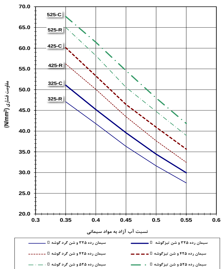
شکل ۷-۶ رابطه نسبت آب به سیمان و مقاومت فشاری در بتن‌های خودتراکم
