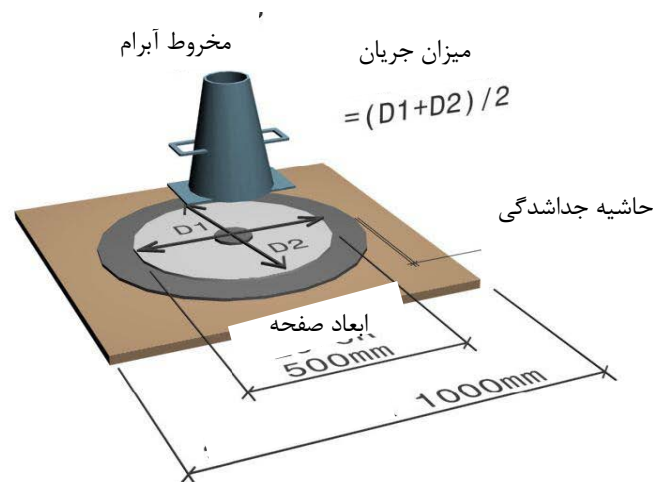
شکل ۱-۳ مشخصات ابزار و وسایل اندازه‌گیری جریان اسلامپ
