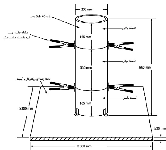
شکل ۳-۸ دستگاه ستون جداسدگی ایستایی مطابق استاندارد ملی ایران ۱۲۲۵۵
