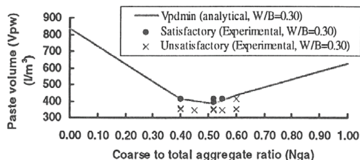
شکل ۴-۱ منحنی تعیین حداقل حجم خمیر در روش حداقل حجم خمیر سیمان
