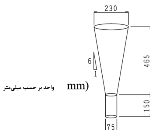
شکل ۷-۳ دستگاه قیف O شکل [58]
