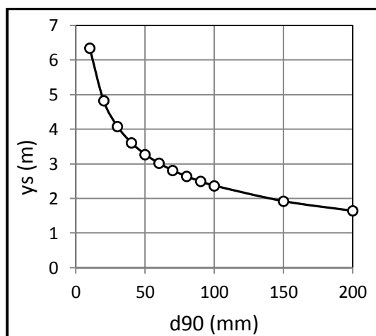
ب- تأثیرپذیری عمق فرسایش از اندازه دانه‌های بستر
