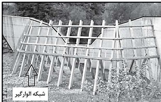
ب- نمونه‌ای از شبکه الوارگیر در بالادست سد رسوبگیر
