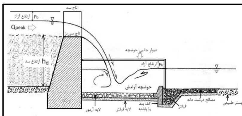
الف- لایه آرمور در حوضچه آرامش و پوشش سنگی در پایین‌دست گف‌بند
