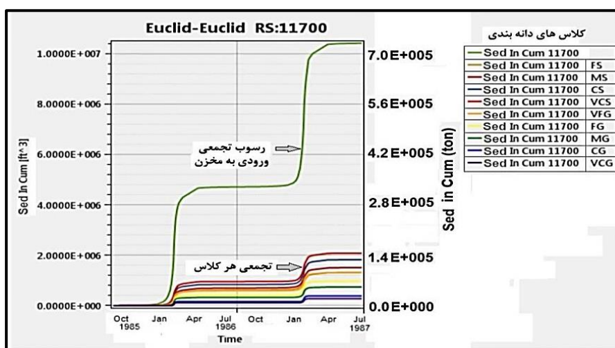
الف - تغییرات زمانی رسوب ورودی به مخزن سد رسوبگیر شکاف‌دار برای محدوده‌های مختلف دانه‌بندی
