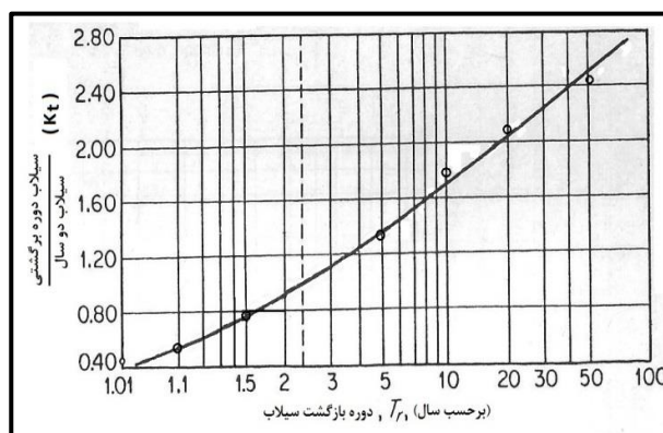
الف- منحنی دوره بازگشت منطقه‌ای برای تعیین سیلاب‌ها
