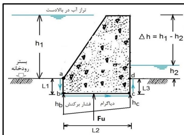
شکل ۴-۱۳- دیاگرام فشار برکنش در پی سازه با استفاده از روش خزش [۷۵، ۱۴]
