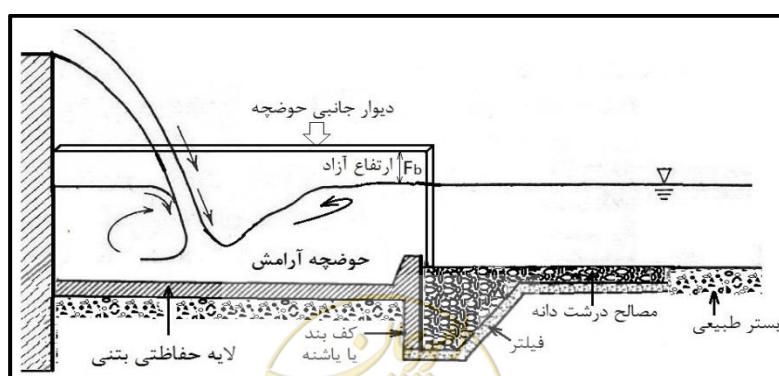
ب- پوشش بتنی در حوضچه آرامش و پوشش سنگی در پایین‌دست گف‌بند
