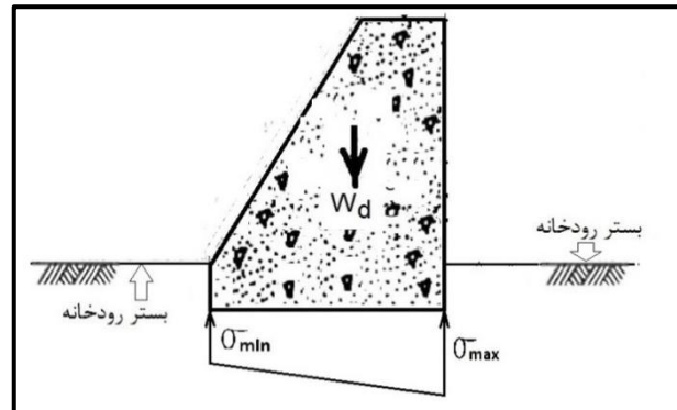
الف- حالت ۱، شرایط بعد از اجرای طرح
