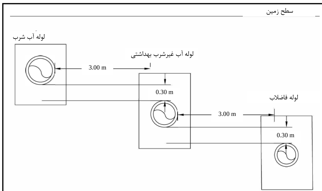
شکل ۲-۵- فاصله توصیه شده لوله آب غیرشرب بهداشتی از لوله‌های آب شرب و فاضلاب
