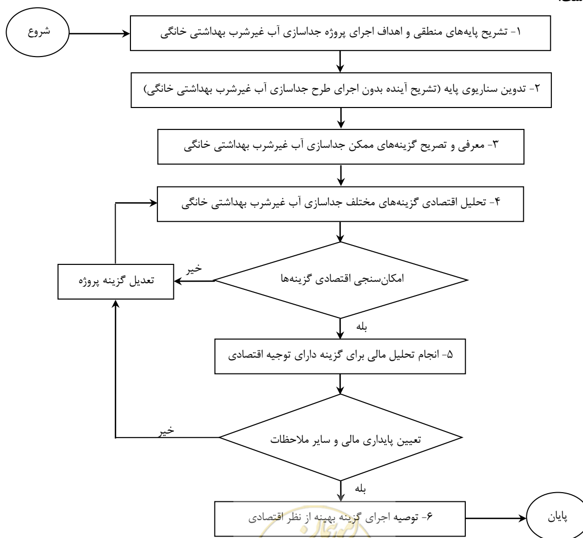
شکل ۳-۲- مراحل بررسی‌های اقتصادی و مالی پروژه‌های جداسازی آب شرب از آب غیرشرب بهداشتی خانگی
